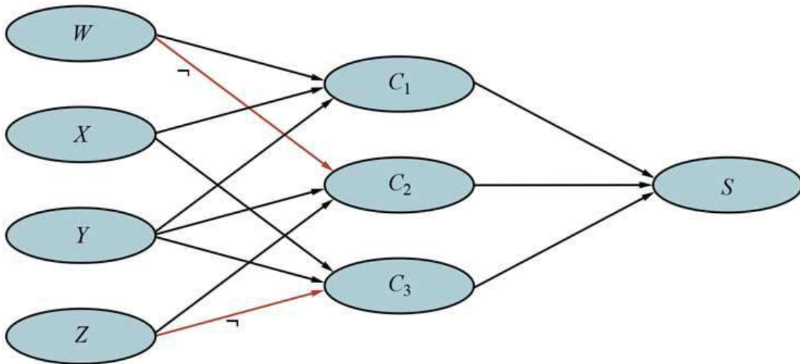
Bayes net encoding of the 3-CNF sentence (W \vee X \vee Y) \wedge (\neg W \vee Y \vee Z) \wedge (X \vee Y \vee \neg Z) .
